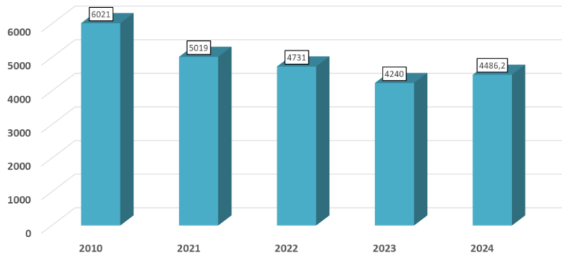
Évolution des consommations de chauffage sur réseaux de chaleur urbain (MWh)
